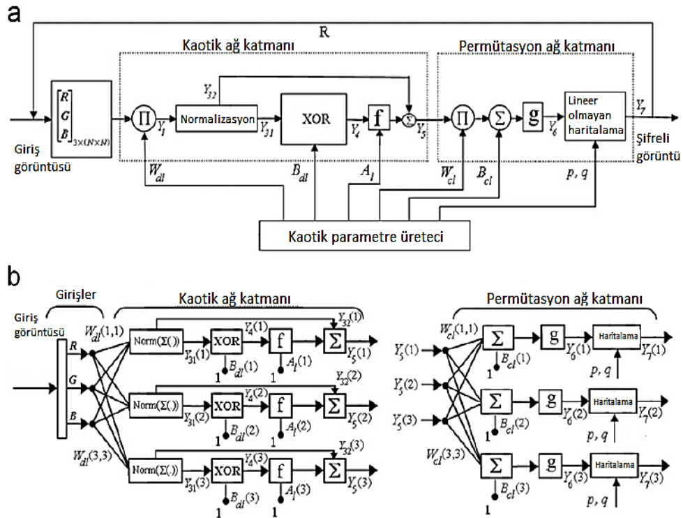
Şekil 4.1. Şifreleme süreci (a) öbek şeması, (b) ağ şeması (Bigdeli, vd., 2012).
