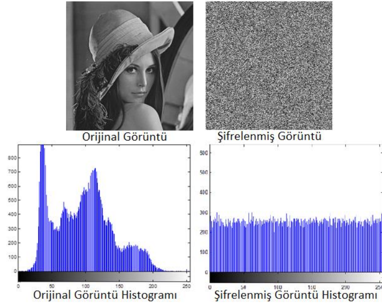
Şekil 5.2. 256x256 orijinal ve şifrelenmiş görüntüye ait histogramlar.
