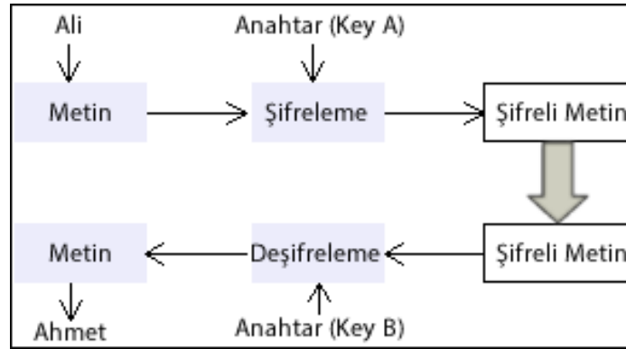
Şekil 2.1. Asimetrik şifreleme yapısı.
