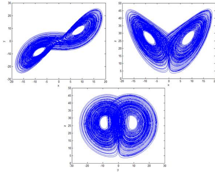
Şekil 3.7. Lorenz sistemine ait x-y, x-z, y-z fazları.
