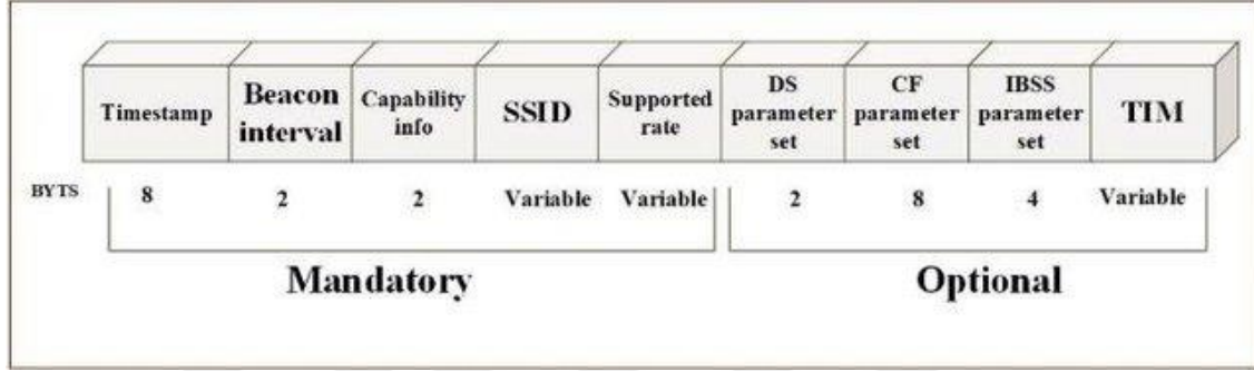
Şekil 2.9. İşaret çerçevesinin vücut kısmı
