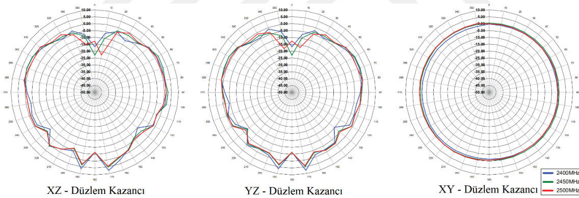
Şekil 3.15. ANT-DB1-LCD-ccc antenin düzlem kazanç değerleri
