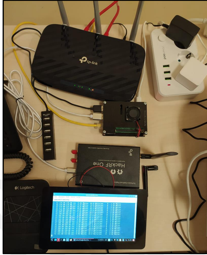
Şekil 3.9. Veri toplama sistemi (ilk hal)
