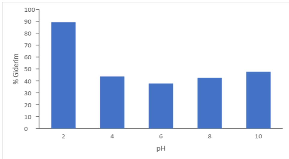
řekil 3.3. Amberlyst A21 ile Remazol Brilliant Blue R’nin % giderimi üzerine pH etkisi ( C_0 : 100 ppm, t : 25 °C, m : 0,05 g, V : 0,05 L, Temas süresi:150 dakika).
