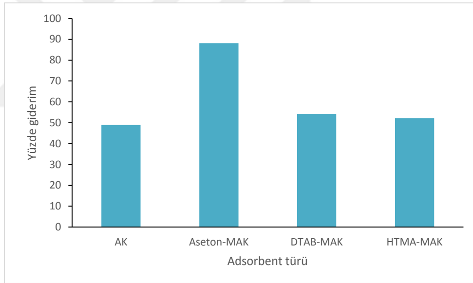
Şekil 3.4. Aktif karbon ile Remazol Brilliant Blue R'nin % giderimi üzerine modifikasyon türünün etkisi ( C_o : 100 ppm, t: 25 °C, m: 0,05 g, V: 0,05 L, Temas süresi: 60 dakika).
